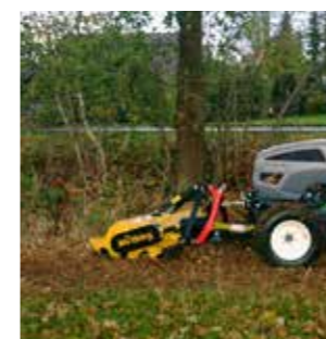
Le MU-C pour montage frontal : points de couplage bas et un boîtier surbaissé (vitesse monorapport de 1.000 ou 2.000 tr/min).
