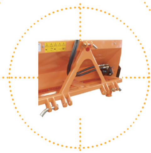
Attelage 3 points tracteur catégorie 0 et 1
