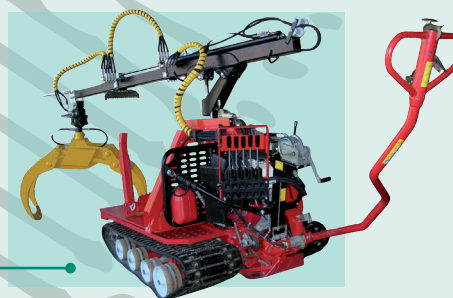
Traineau Sulky.
